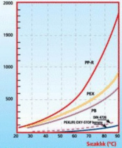
Bazı plastik boruların oksijen geçirgenlik özellikleri
